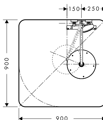
Instalacja w strefie prysznica
